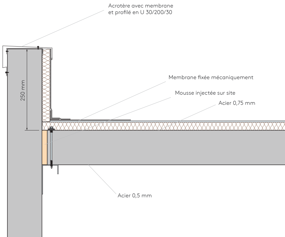
Figure 4 - Détail d'utilisation pour toiture plane avec complément d'isolation et membrane PVC fixée mécaniquement
