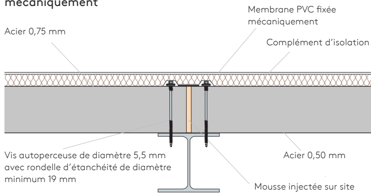
Figure 3 - Détail d'utilisation pour toiture plane avec complément d'isolation et membrane PVC fixée mécaniquement
